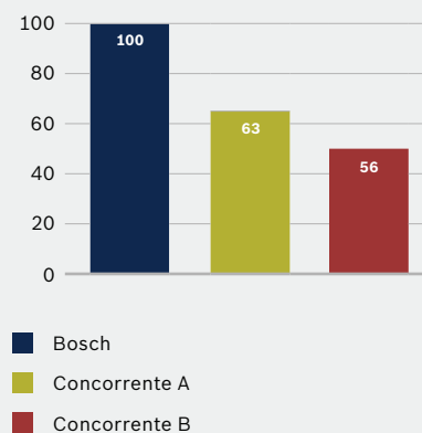
Prestazioni di scalpellatura nel calcestruzzo C 20/25
